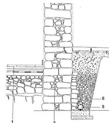
Sistema drenante verticale per murature parzialmente interrate
