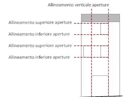
Allineamento tipo delle forometrie in una unità edilizia monocellulare
