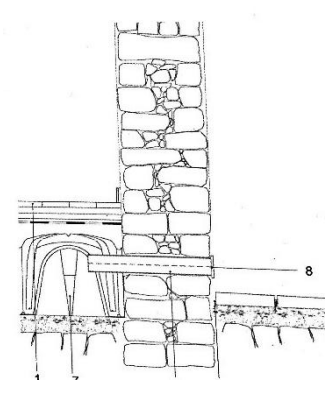
Sistema drenante con casseri prefabbricati
