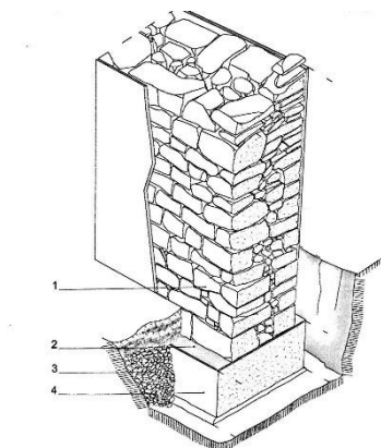
Realizzazione di nuova sottofondazione
