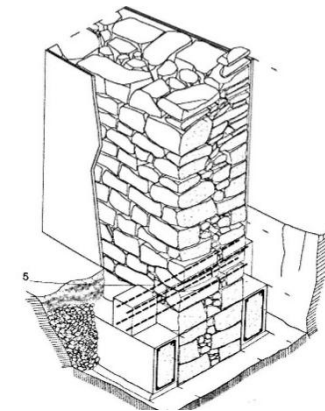
Consolidamento mediante cordoli armati collegati tra loro 5_ elementi in calcestruzzo armato per il collegamento dei due cordoli alla muratura esistente
