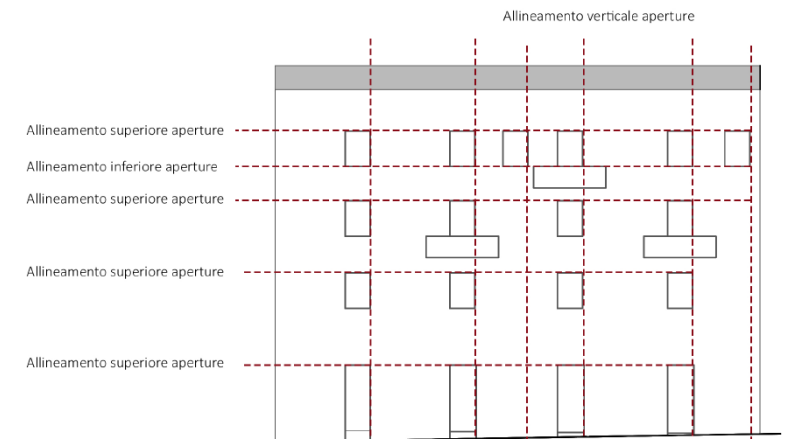
Allineamento tipo delle forometrie in una unità edilizia pluricellulare
